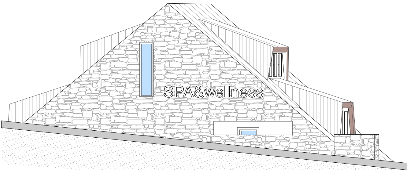
ИЗГЛЕД СА ЈУГОИСТОКА R=1:50
