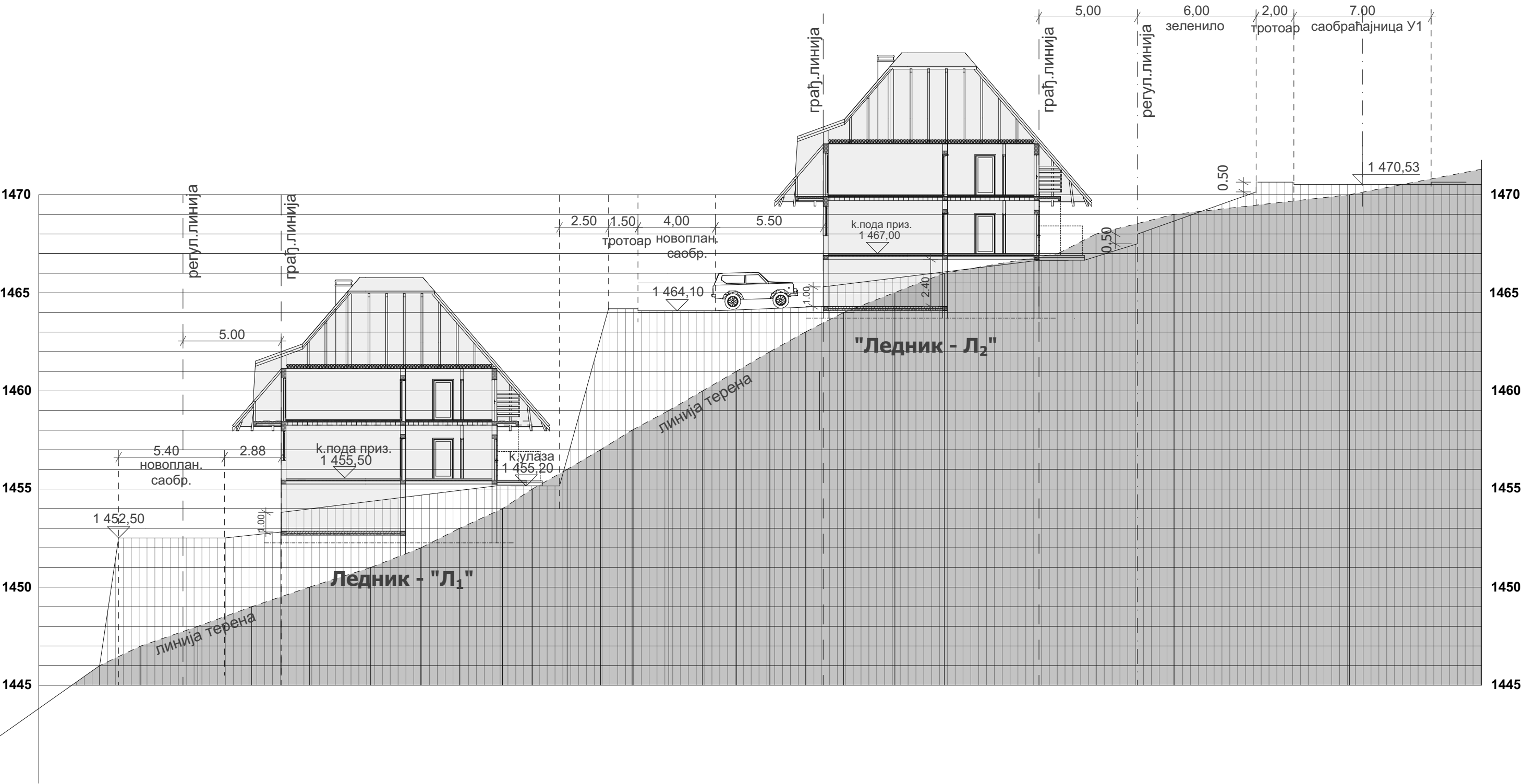
ПРЕСЕК 1-1 КРОЗ ТЕРЕН
